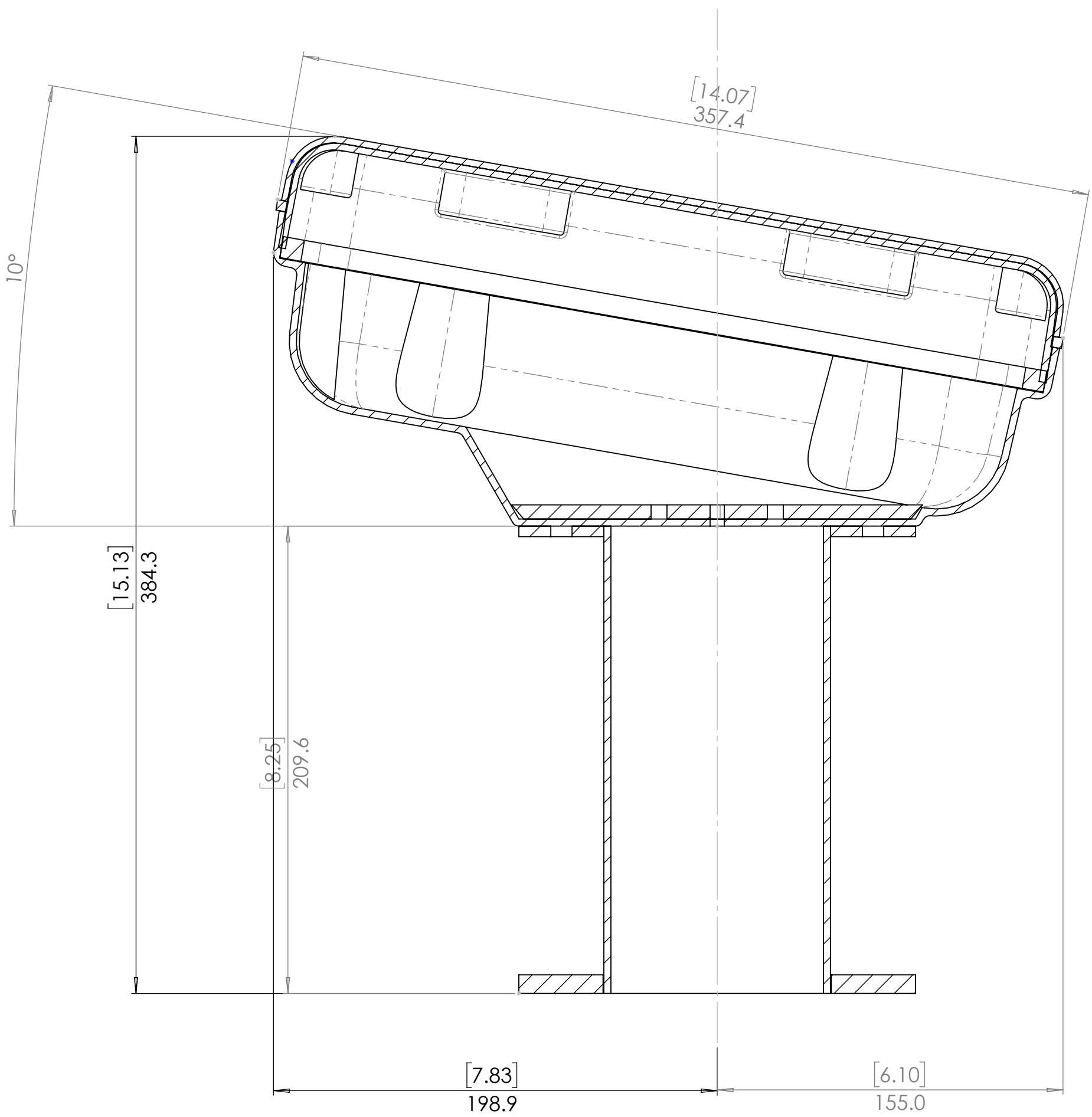
SECTION A-A
